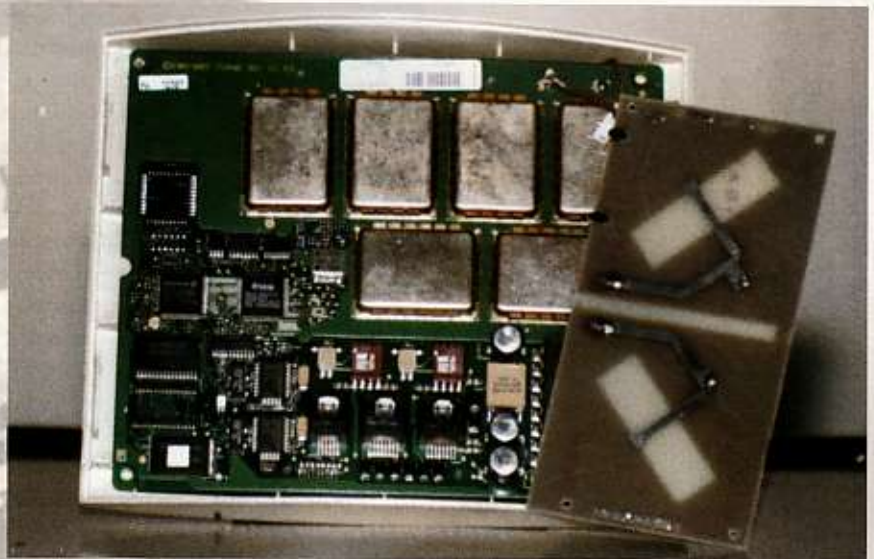
Consumentenbasisstation met polarisation diversity techniek.
